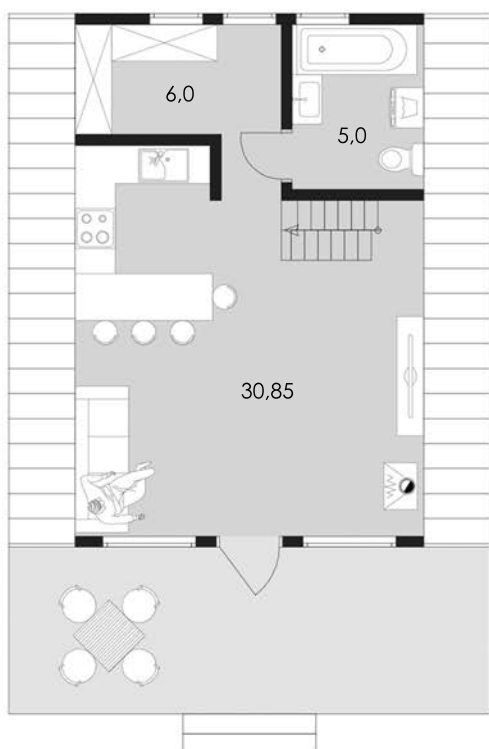
ПОВЕРХОВІ ПЛАНИ
